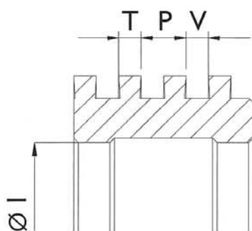
Bloccaggio a pacco Free locking
