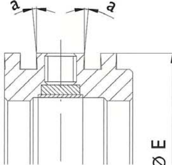
Bloccaggio multilock Multilock
