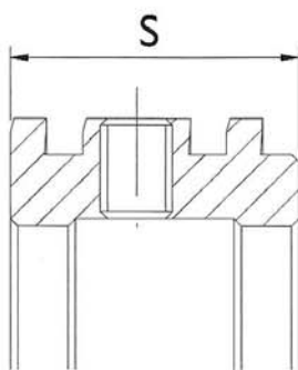
Bloccaggio con grano Grub screw locking
